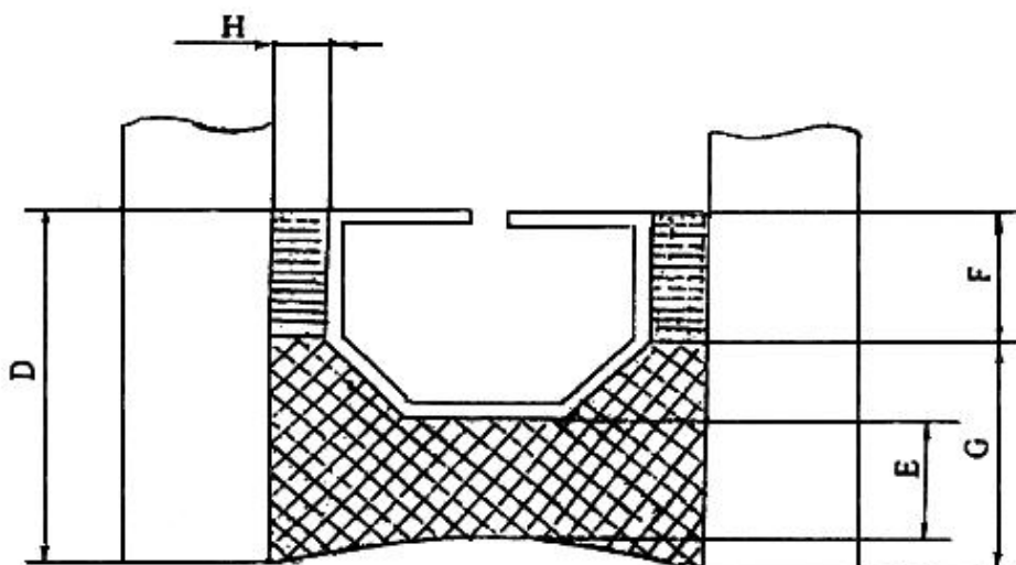
Рисунок 2 - Герметизирующие слои стеклопакета
