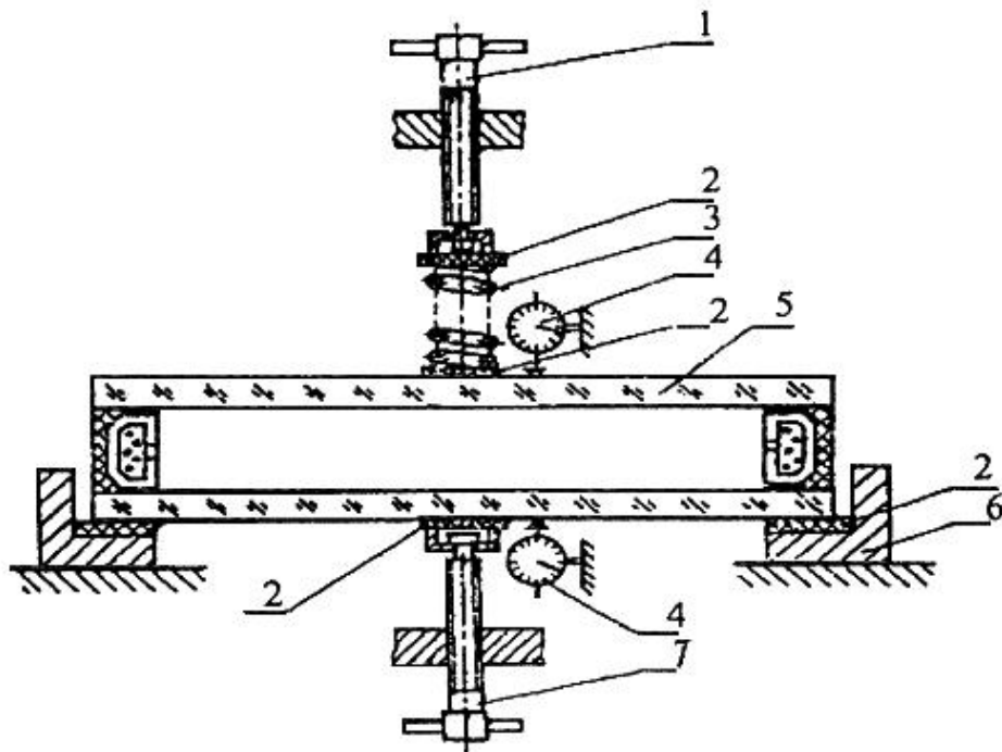
Рисунок 6 - Схема стенда для проверки герметичности
